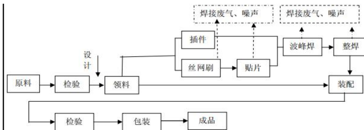
图 1-1 生产工艺流程与产污图
