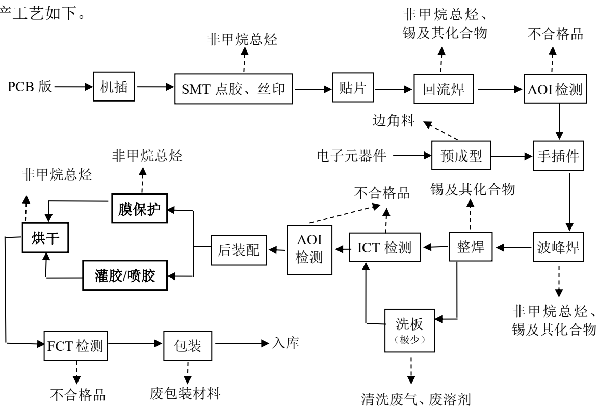
图 5-1 生产工艺流程与产污图
